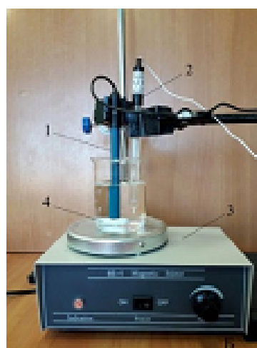
Рис. 2. Установка для определения концентрации (активности) хлорид-ионов в растворе. А: 1 — корпус датчика для определения Cl - -ионов; 2 — разъем Micro USB для подключения к компьютеру; 3 — разъем BNC для подключения рабочего электрода; 4 — разъем для подключения электрода сравнения. Б: 1 — ионоселективный электрод (рабочий электрод); 2 — электрод сравнения (хлорсеребряный электрод); 3 — магнитная мешалка; 4 — якорь магнитной мешалки
