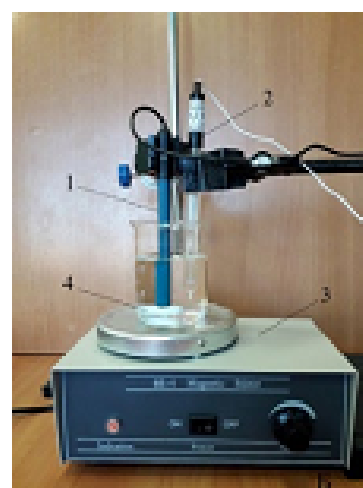
Рис. 2. Установка для определения концентрации (активности) хлорид-ионов в растворе. А: 1 — корпус датчика для определения \text{Cl}^- -ионов; 2 — разъем Micro USB для подключения к компьютеру; 3 — разъем BNC для подключения рабочего электрода; 4 — разъем для подключения электрода сравнения. Б: 1 — ионоселективный электрод (рабочий электрод); 2 — электрод сравнения (хлорсеребряный электрод); 3 — магнитная мешалка; 4 — якорь магнитной мешалки
